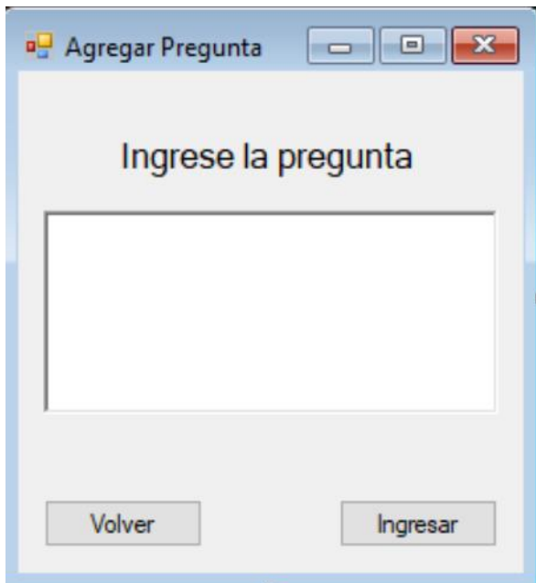
Ilustración 30 Agregar pregunta
