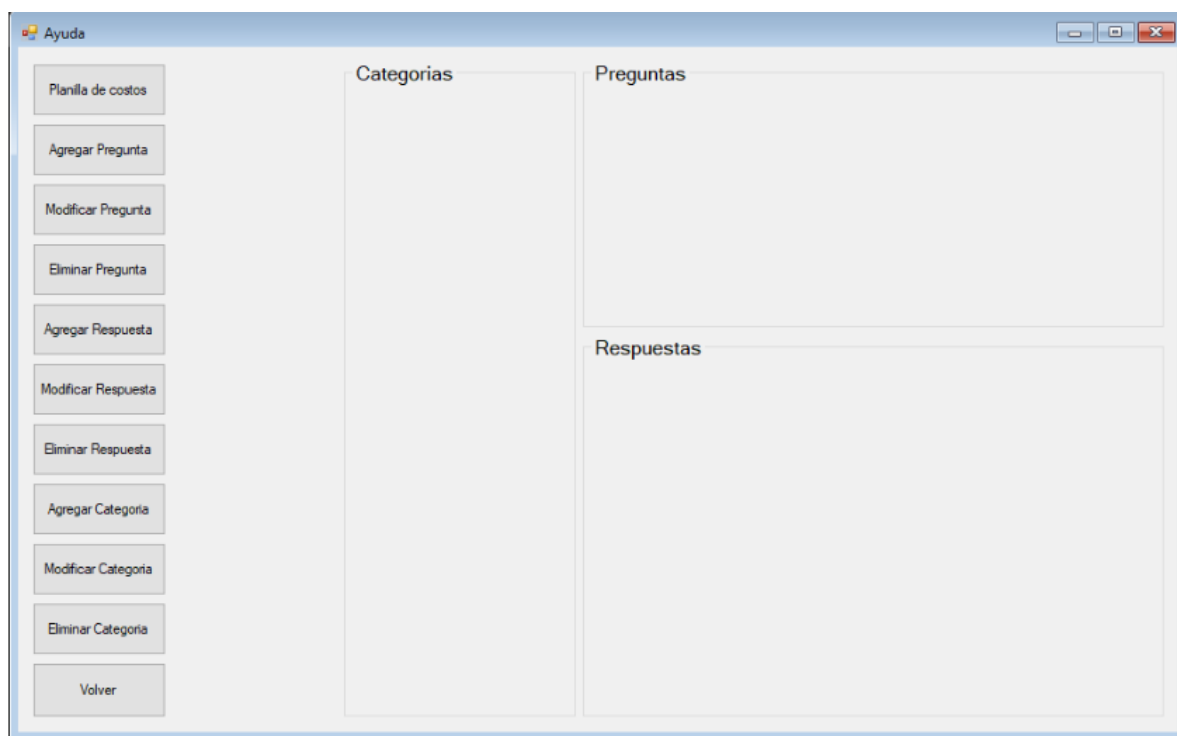
Ilustración 26 Ayuda
