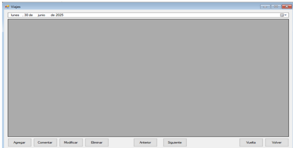
Ilustración 6 Viajes
