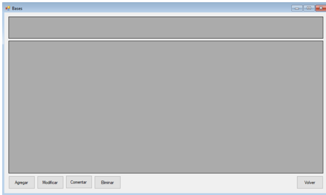
Ilustración 12Bases
