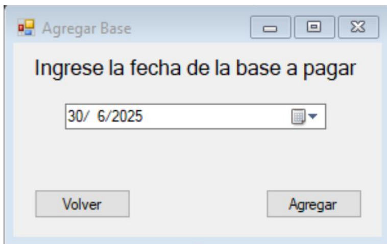
Ilustración 13Agregar base
