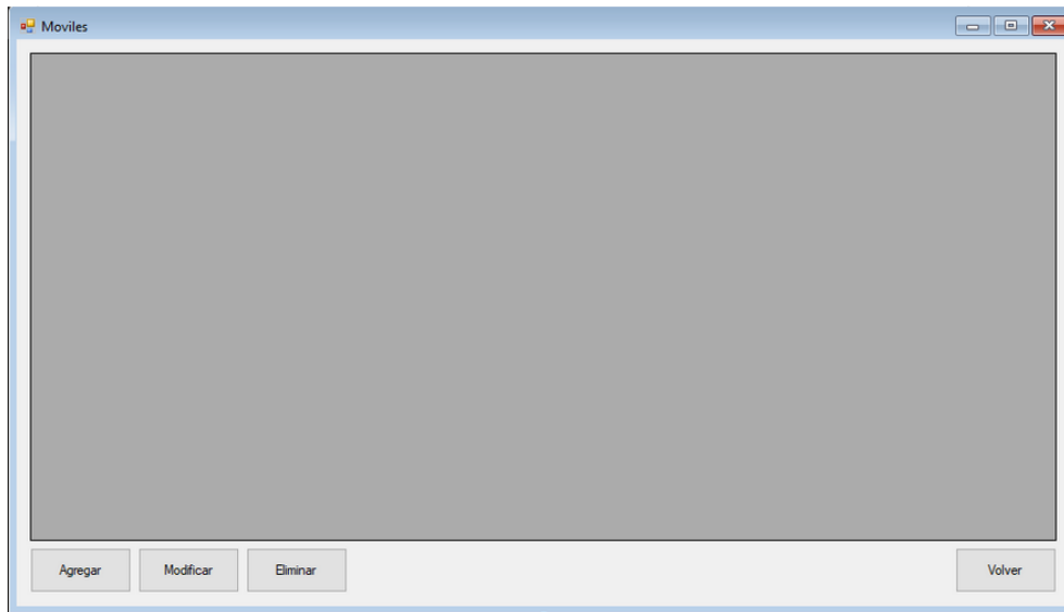
Ilustración 21Móviles
