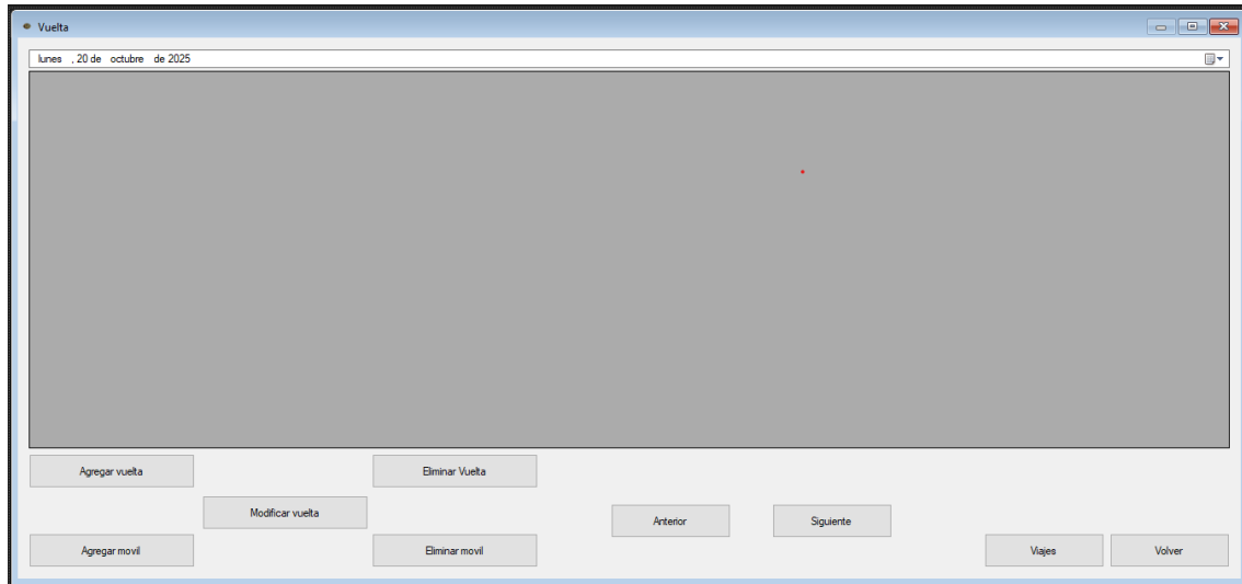
Ilustración 10Vuelta
