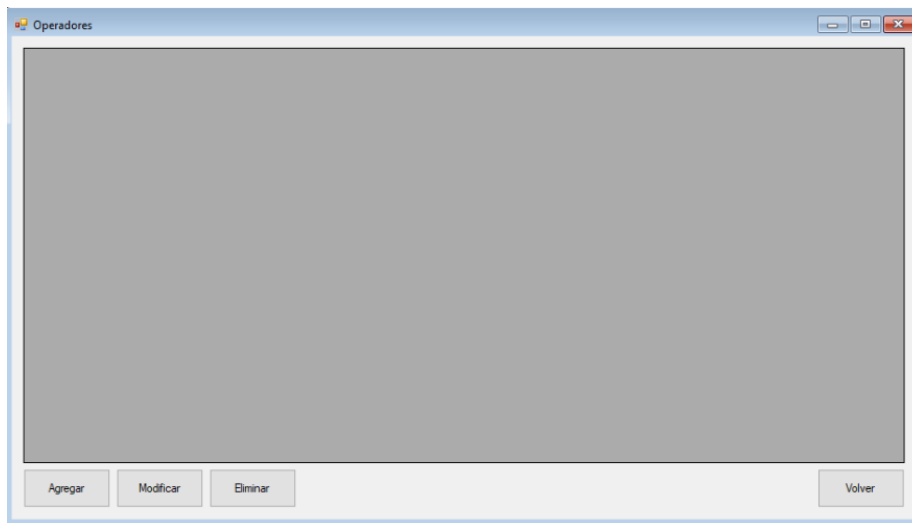
Ilustración 17 Operadores
