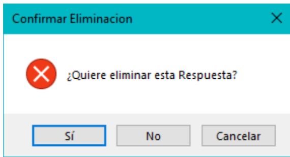
Ilustración 35 Eliminar respuesta
