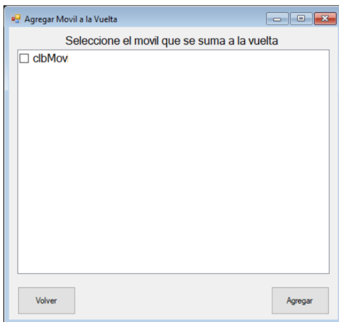
Ilustración 11Agregar vuelta
