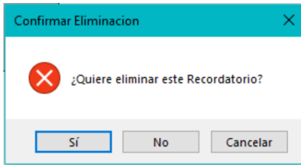
Ilustración 5 Eliminar inicio
