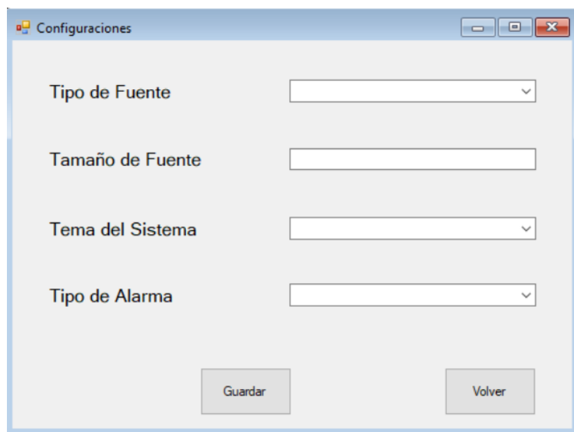
Ilustración 25 Configuraciones
