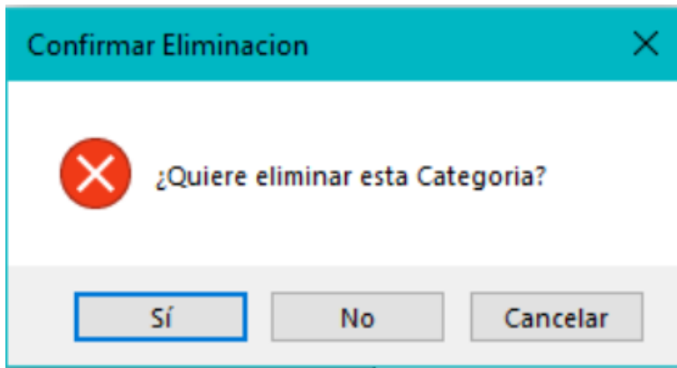
Ilustración 29 Eliminar categoría
